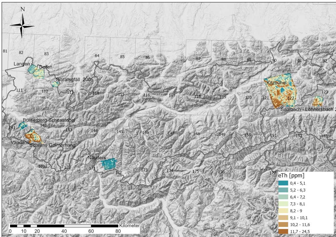
Abbildung 6: Darstellung der interpolierten Thorium Konzentrationen aus dem Datensatz radiometrie_2009_Vbg_Tir_Sbg_BMN_M31.txt ; Hintergrund: © basemap.at (Gelände)
