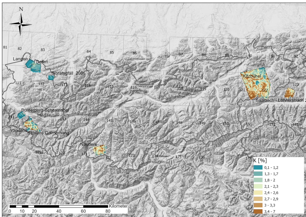
Abbildung 4: Darstellung der interpolierten Kalium Konzentrationen aus dem Datensatz radiometrie_2009_Vbg_Tir_Sbg_BMN_M31.txt ; Hintergrund: © basemap.at (Gelände)
