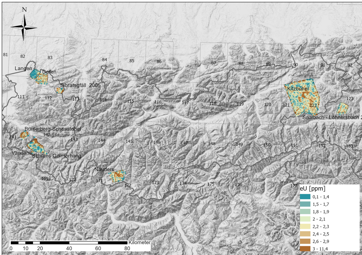
Abbildung 5: Darstellung der interpolierten Uran Konzentrationen aus dem Datensatz radiometrie_2009_Vbg_Tir_Sbg_BMN_M31.txt , Hintergrund: © basemap.at (Gelände)
