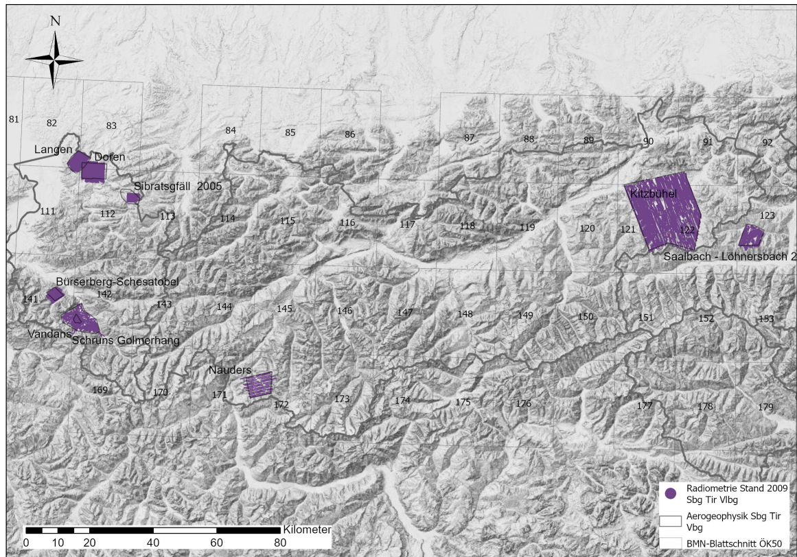
Abbildung 3: Verteilung der Messdaten und Lage der Fluggebiete, die im Datensatz radiometrie_2009_Vbg_Tir_Sbg_BMN_M31.txt enthalten sind. Details zu den jeweiligen Fluggebieten sind Tabelle 1 bzw. den darin zitierten Projektberichten zu entnehmen. Hintergrund: © basemap.at (Gelände)
