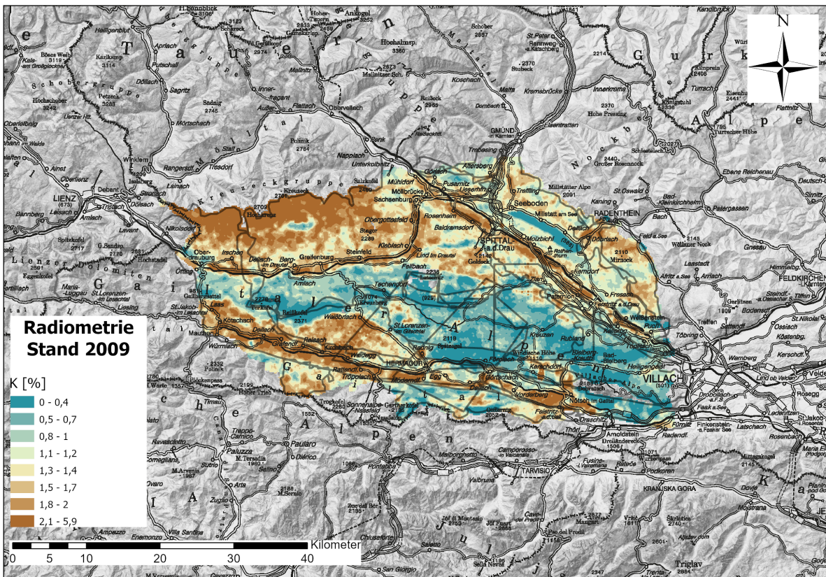
Abbildung 4: Darstellung der interpolierten Kalium Konzentrationen aus dem Datensatz radiometrie_2009_Ktn_BMN_M31.txt ; Hintergrund: © basemap.at (Gelände)
