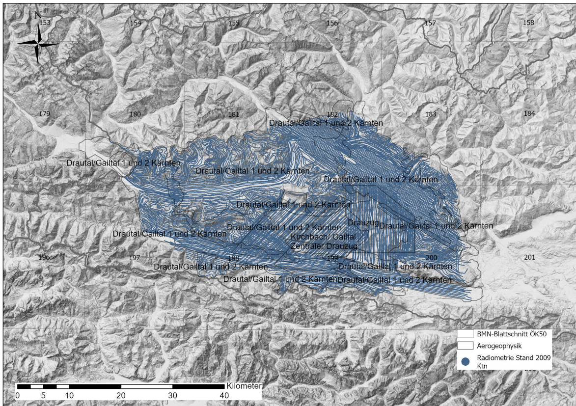
Abbildung 3: Verteilung der Messdaten und Lage der Fluggebiete, die im Datensatz radiometrie_2009_Ktn_BMN_M31.txt enthalten sind. Details zu den jeweiligen Fluggebieten sind Tabelle 1 bzw. den darin zitierten Projektberichten zu entnehmen. Hintergrund: © basemap.at (Gelände)
