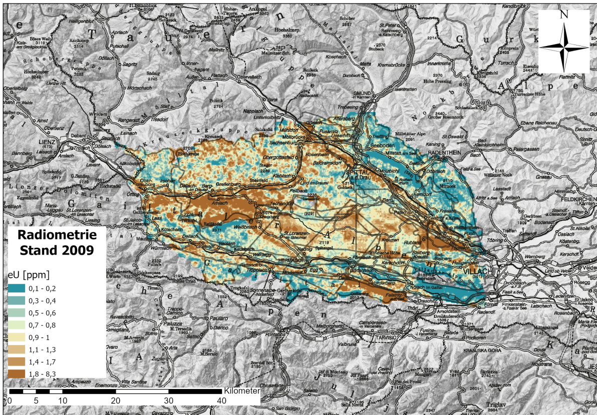
Abbildung 5: Darstellung der interpolierten Uran Konzentrationen aus dem Datensatz radiometrie_2009_Ktn_BMN_M31.txt , Hintergrund: © basemap.at (Gelände)
