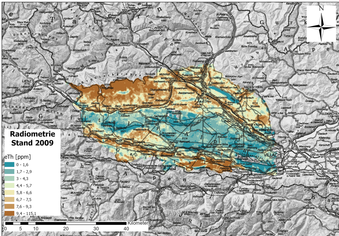
Abbildung 6: Darstellung der interpolierten Thorium Konzentrationen aus dem Datensatz radiometrie_2009_Ktn_BMN_M31.txt ; Hintergrund: © basemap.at (Gelände)
