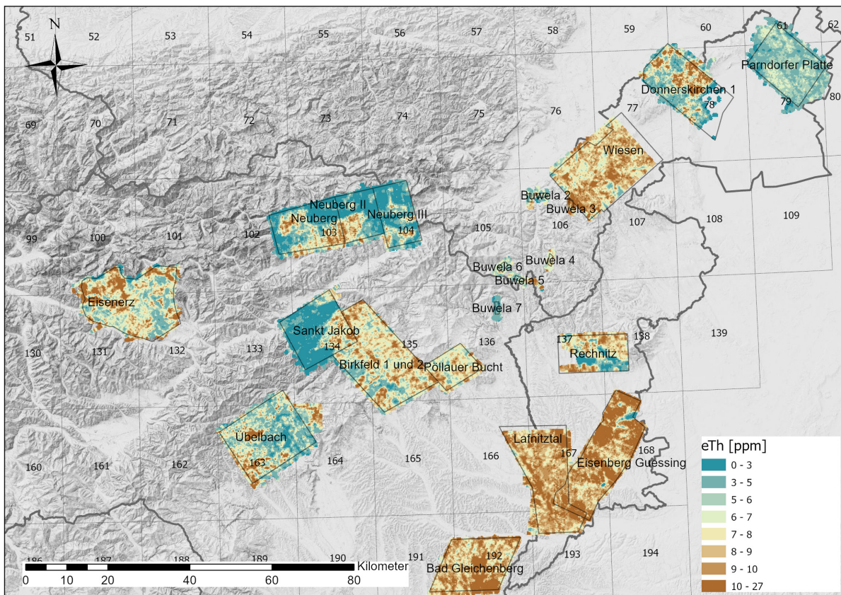
Abbildung 6: Darstellung der interpolierten Thorium Konzentrationen aus dem Datensatz radiometrie_2009_Stmk_Bgld_BMN_M31.txt , Hintergrund: © basemap.at (Gelände)
