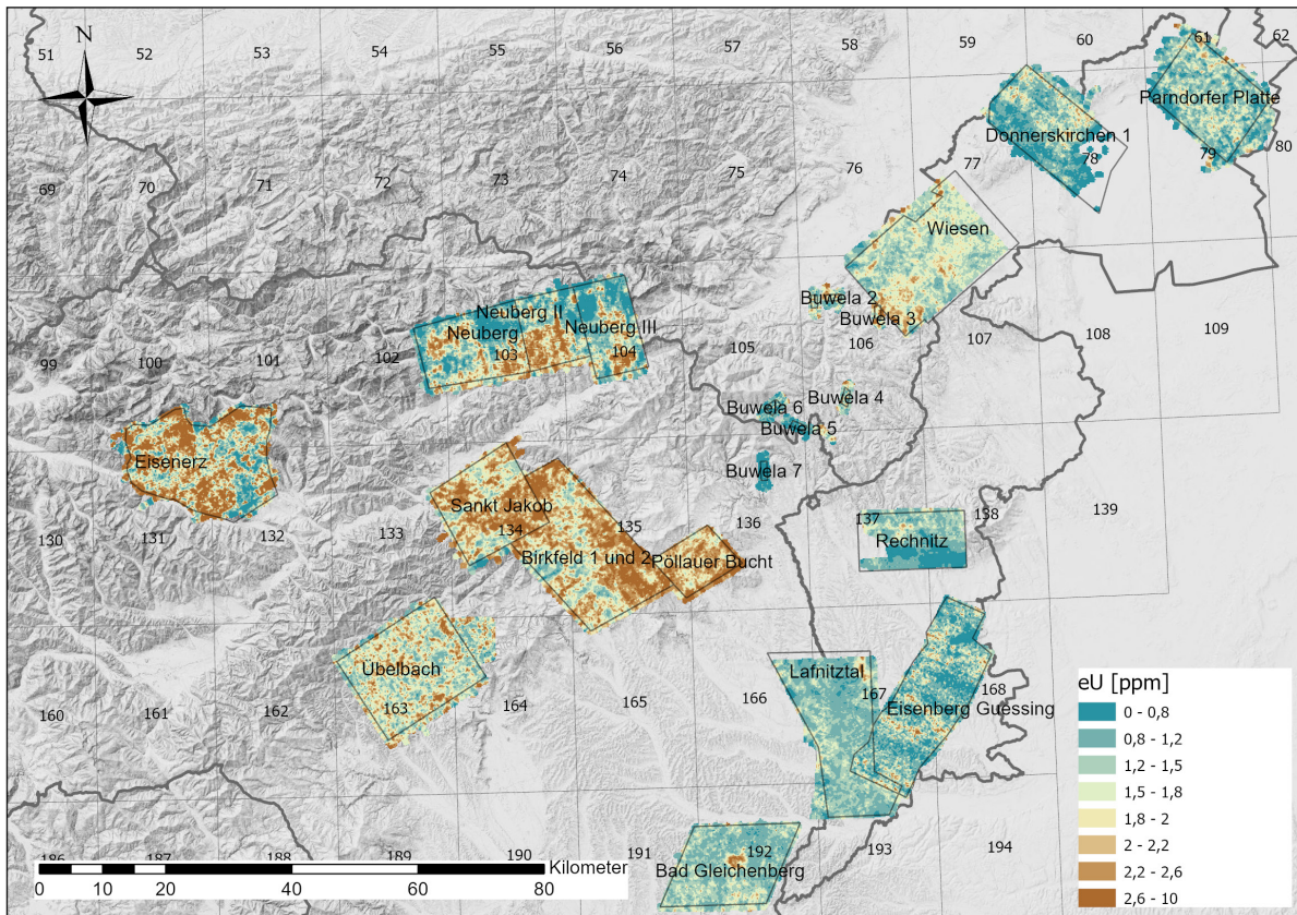
Abbildung 5: Darstellung der interpolierten Uran Konzentrationen aus dem Datensatz radiometrie_2009_Stmk_Bgld_BMN_M31.txt , Hintergrund: © basemap.at (Gelände)
