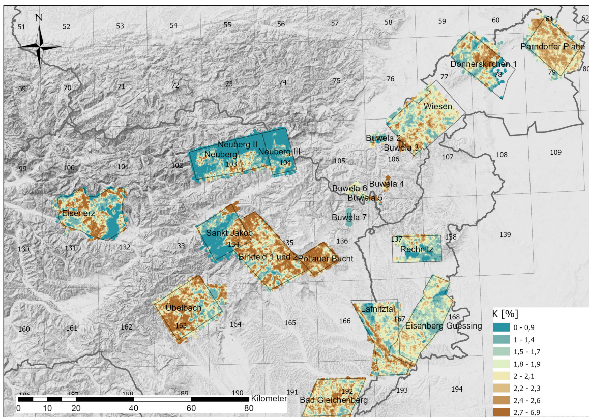
Abbildung 4: Darstellung der interpolierten Kalium Konzentrationen aus dem Datensatz radiometrie_2009_Stmk_Bgld_BMN_M31.txt ; Hintergrund: © basemap.at (Gelände)
