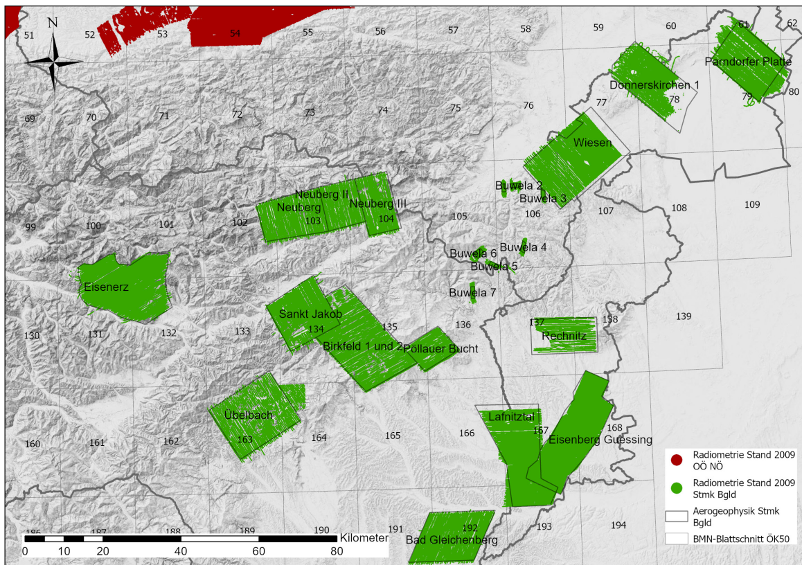
Abbildung 3: Verteilung der Messdaten und Lage der Fluggebiete, die im Datensatz radiometrie_2009_Stmk_Bgld_BMN_M31.txt enthalten sind. Details zu den jeweiligen Fluggebieten sind Tabelle 1 bzw. den darin zitierten Projektberichten zu entnehmen. Hintergrund: © basemap.at (Gelände)
